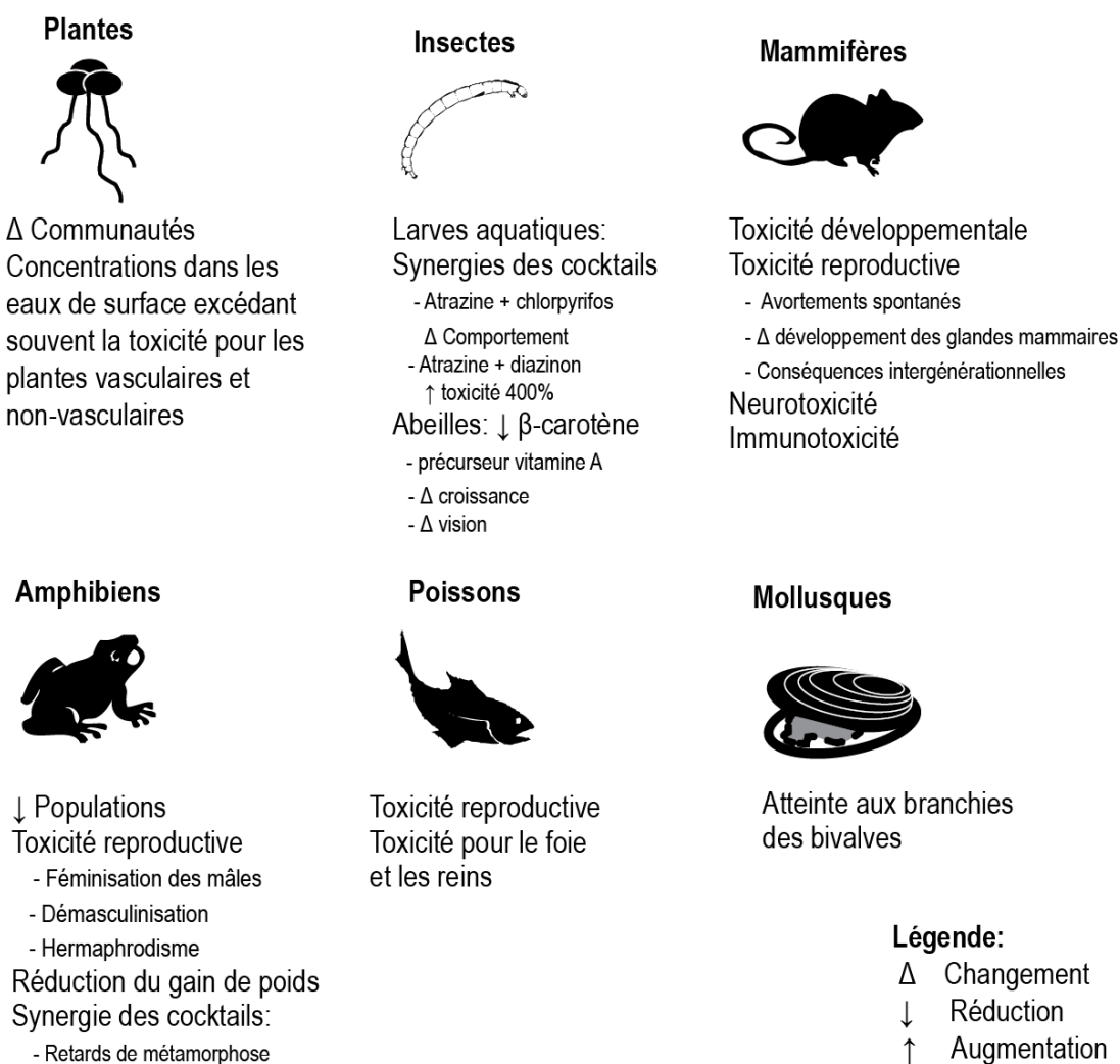
Figure 4 : Écotoxicité de l'atrazine.
